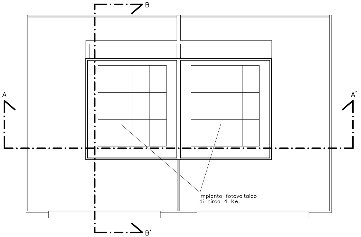
PIANO COPERTURA
